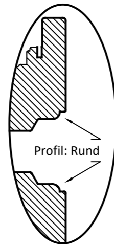
Vertikalsnitt Karmpost
