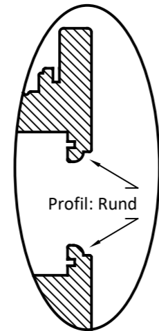
Vertikalsnitt Karmpost
